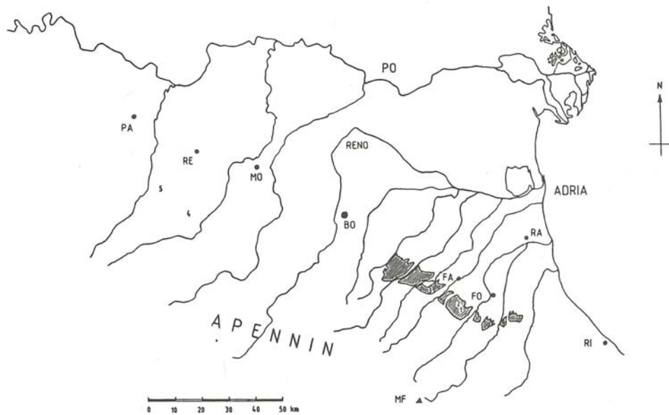
Abb. 3. Übersichtskarte. Schraffiert: pliozän-pleistozäne Tone mit 1 Castrocaro, 2 Torrente Samoggia, 3 Brisighella. In den «argille scagliose» die Standorte 4 Baiso, 5 Canossa. – BO: Bologna, FA: Faenza, FO: Forlì, MF: Monte Falterona, MO: Modena. PA: Parma, RA: Ravenna, RE: Reggio nell'Emilia, RI: Rimini.
